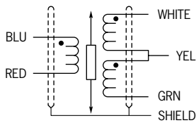
Wiring Schematic
